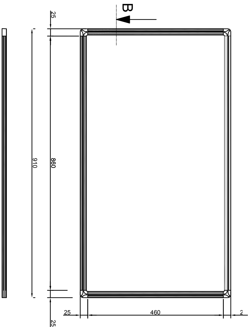
ÖLÇEK 1/1 1/110
