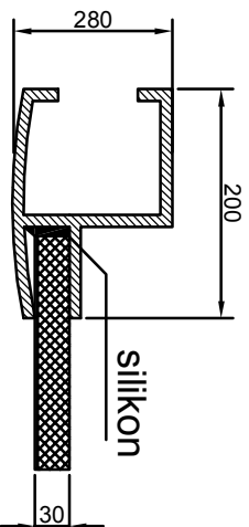
B-DETAYI ÖLÇEK: 1/1
